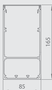
Sezione trave
