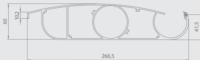
Sezione dell'aletta
