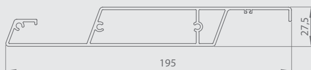
Sezione lamella
